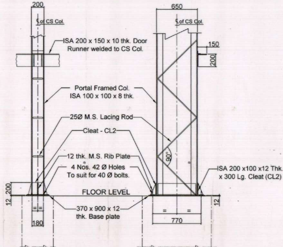
ELEVATION
