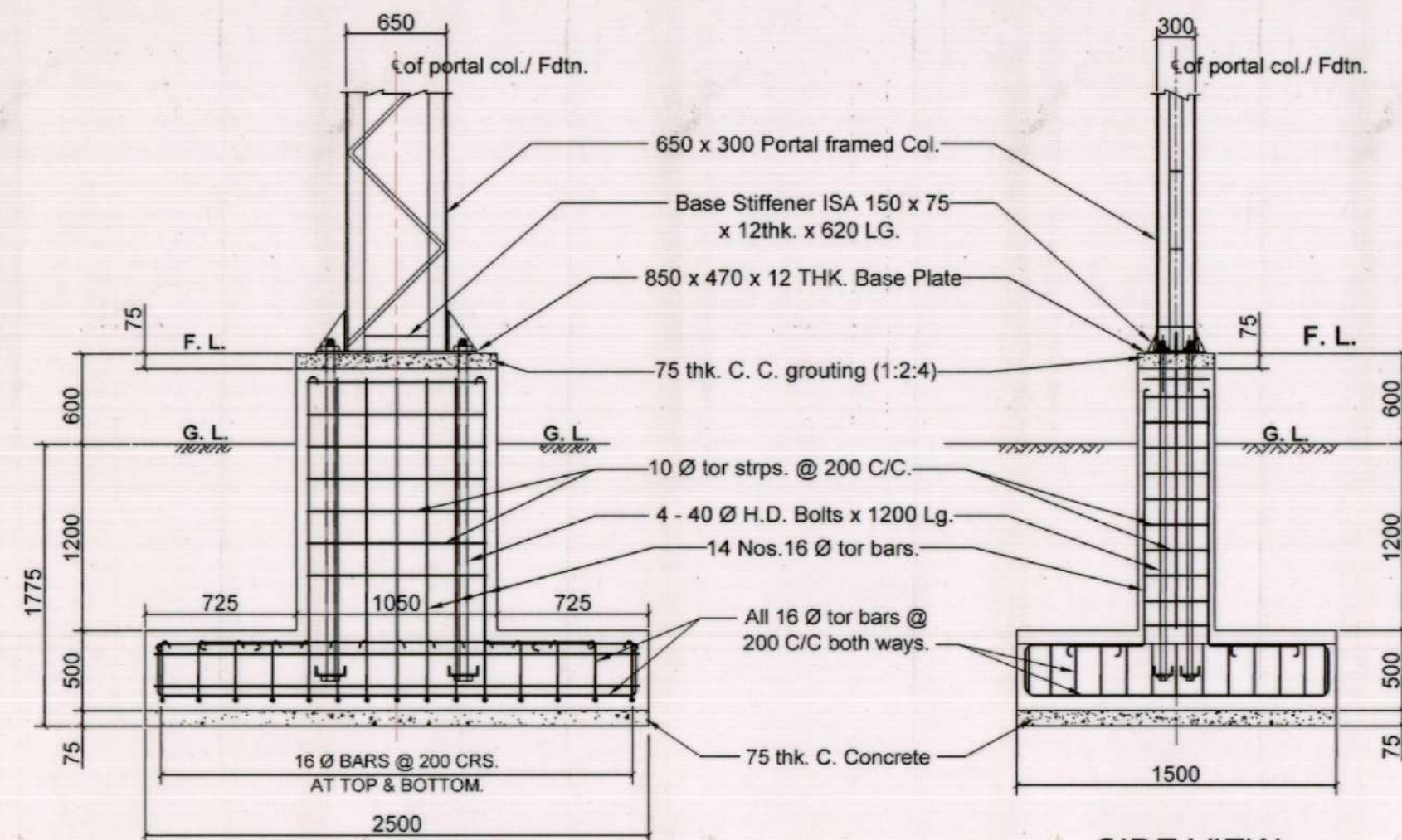
ELEVATION
