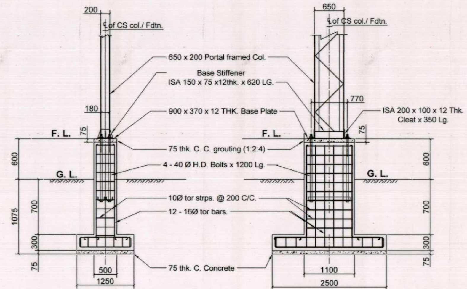
ELEVATION
