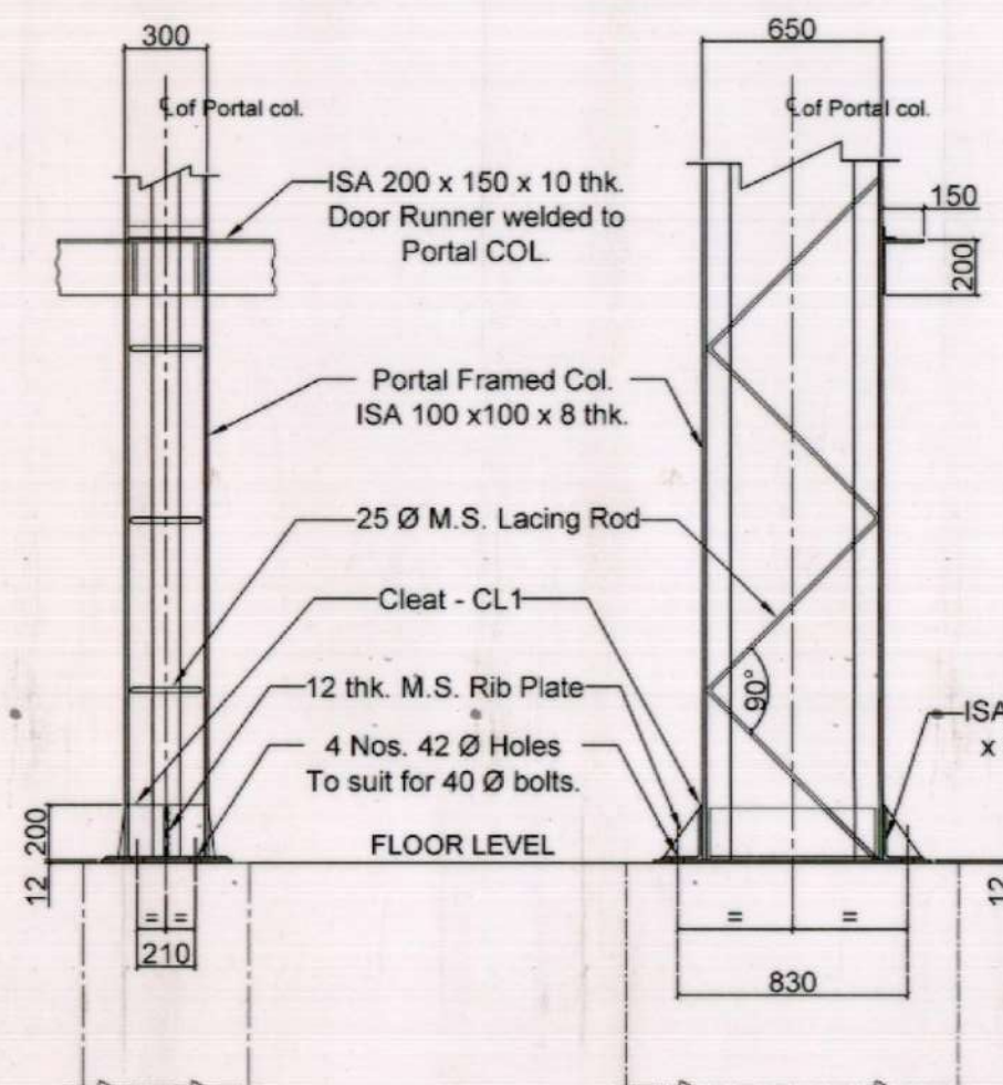
ELEVATION
