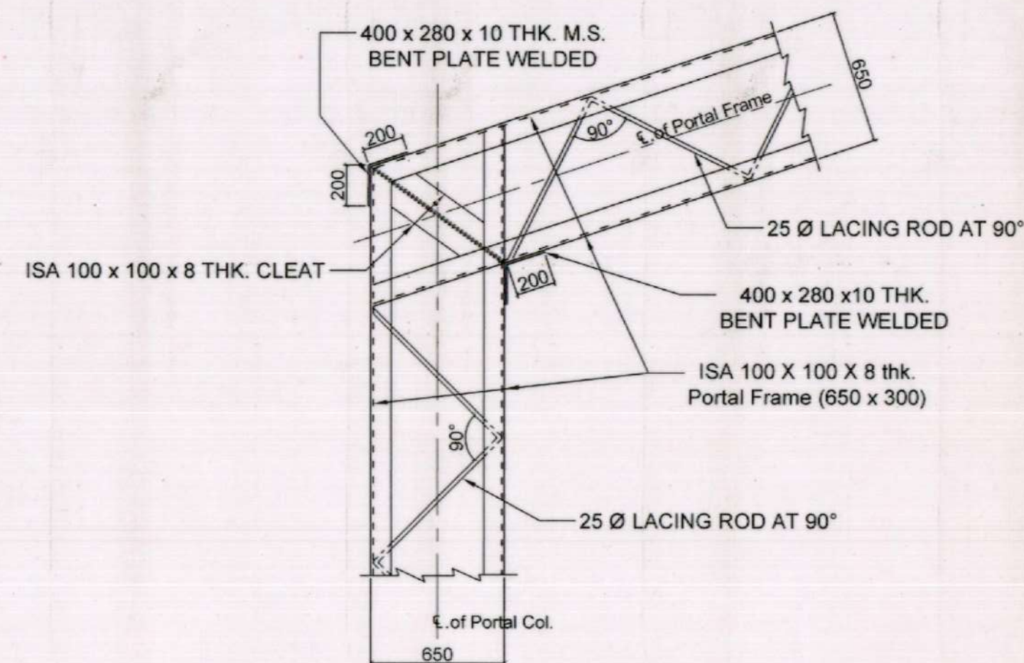
ENLGD. DETAILS AT 'A'
