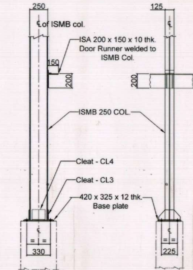
ELEVATION
