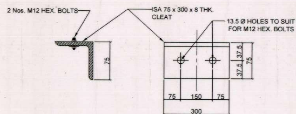
ENLRGD. CLEAT 1
