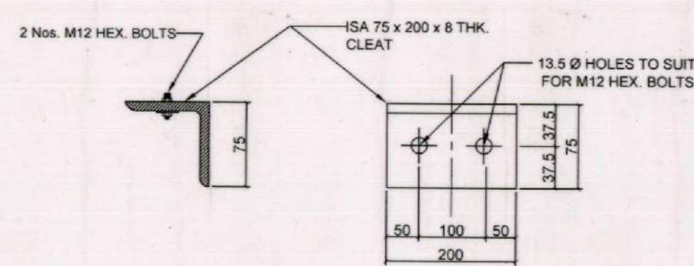
ENLRGD. CLEAT 2
