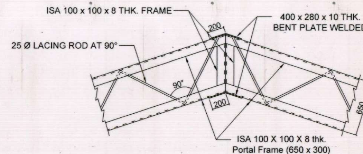
ENLGD. DETAILS AT 'B'
