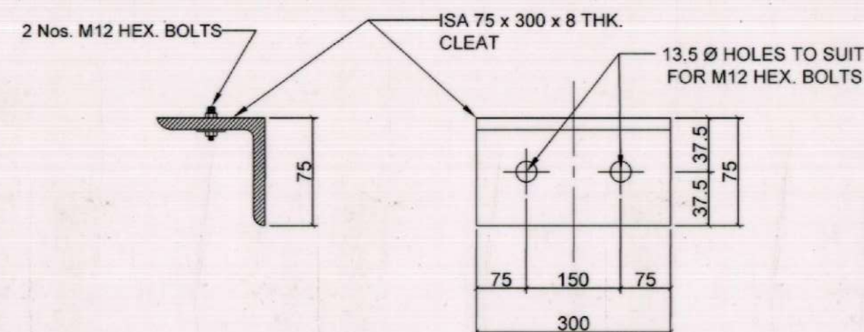
ENLRGD. CLEAT 3
