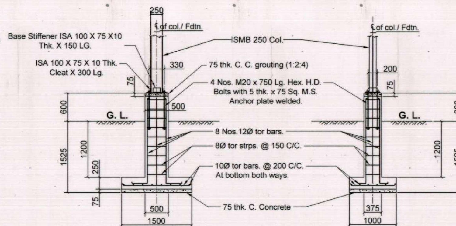
ELEVATION
