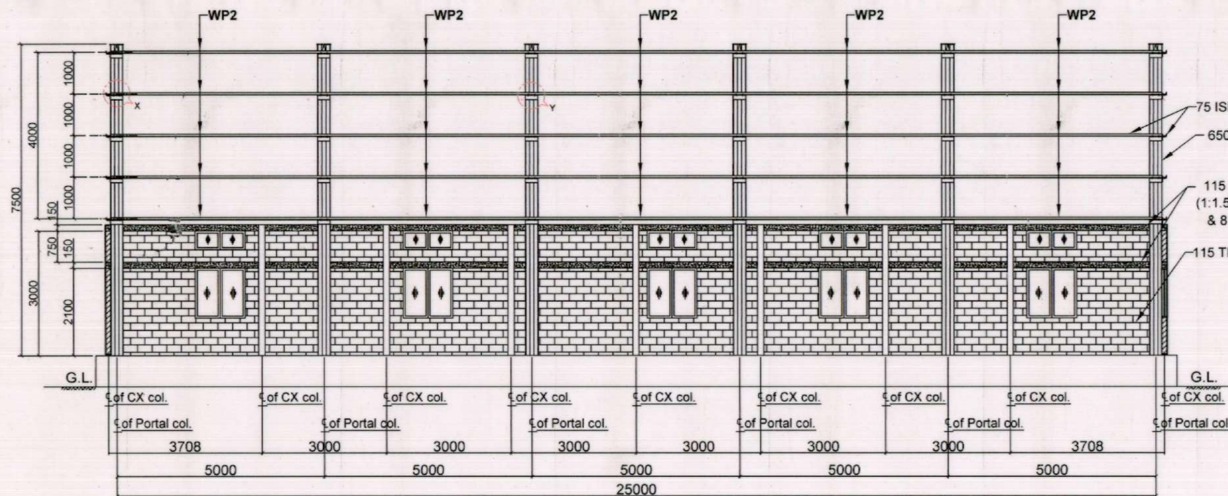
ELEVATION
